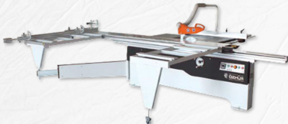
SWN 2200/ SWN 2800 SWN 3200/ SWN 3800 Circular Panel Saw
